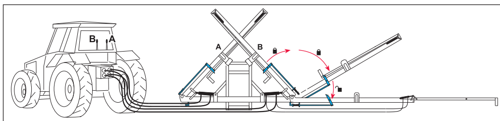
Sistema 8, apertura barra, direttamente dal trattore, mediante 2 distributori doppio effetto Sistema 8, Boom Unfolded Directly By 2 Double Effect Hydraulic Distributors of the Tractor
