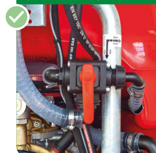
Agitateur (désactivable)
