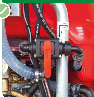
Agitateur (désactivable)
