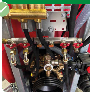
Barre de distribution
