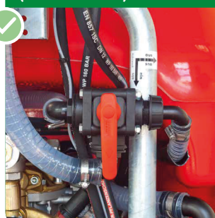
Agitateur (désactivable)
