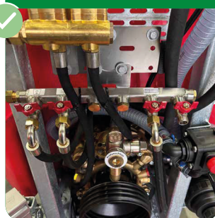
Barre de distribution
