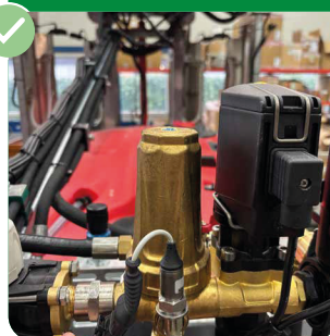
Filtre sous pression
